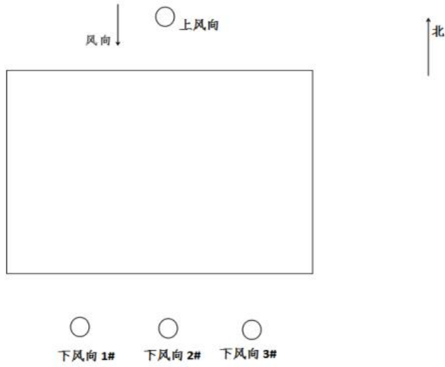
北风时无组织废气检测布点图
