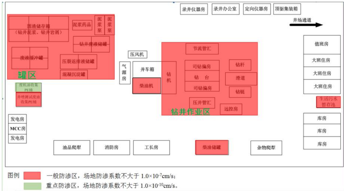
井场防渗示意图
