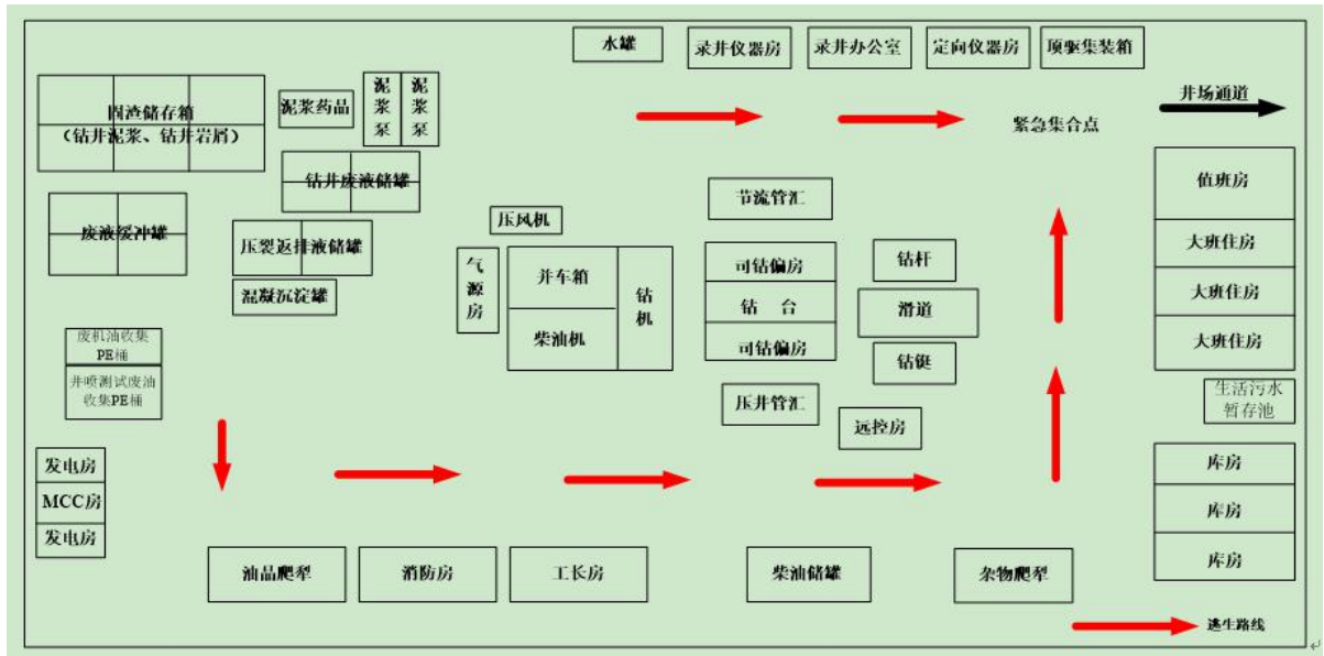
井场布置图
