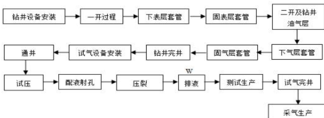
图 1-1 钻井工艺流程图
