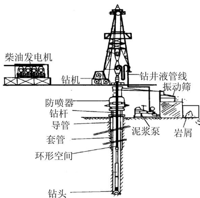
钻井作业示意图
