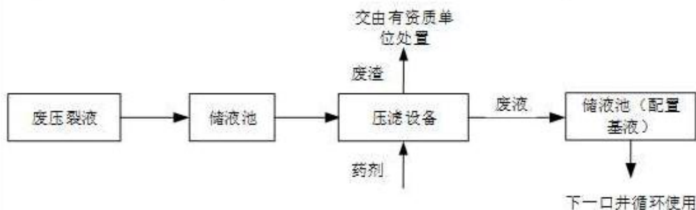
废压裂液处理工艺流程图
