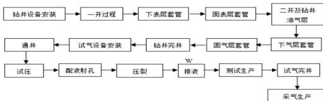
图 1-1 钻井工艺流程图
