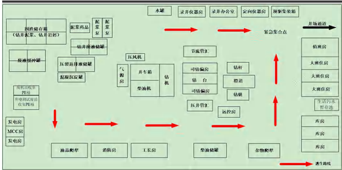
施工期采气井场平面布置示意图
