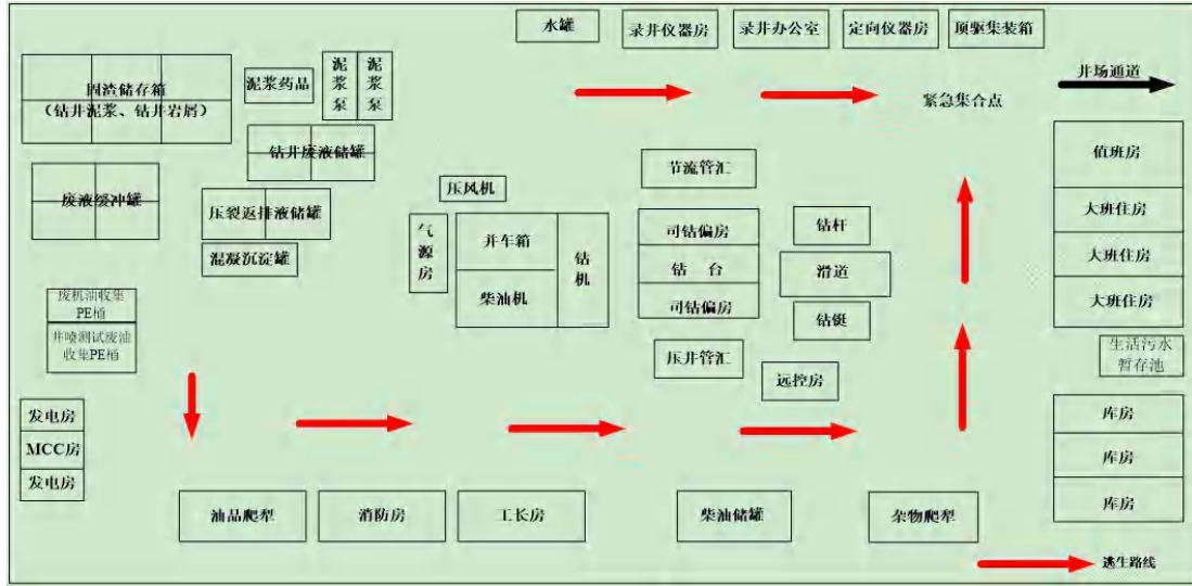
施工期采气井场平面布置示意图
