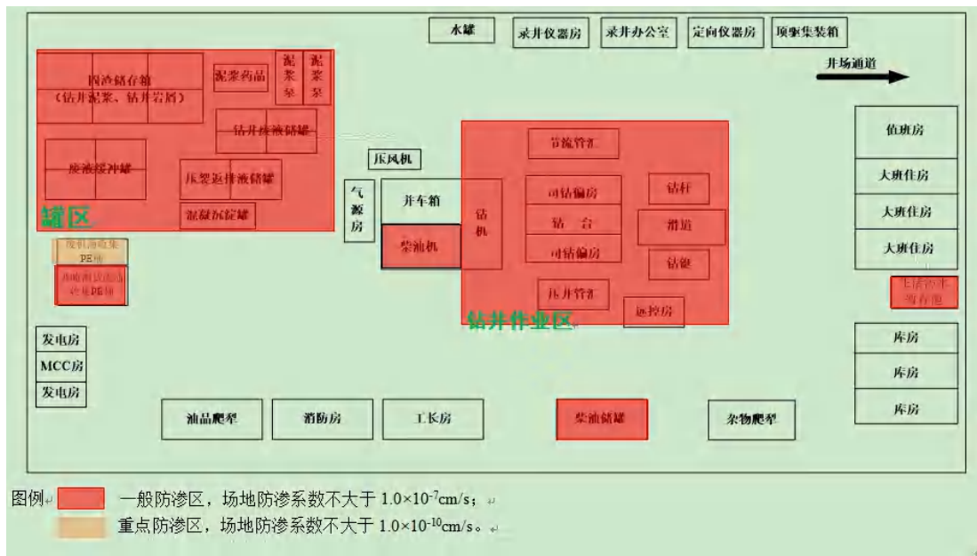
施工场地防渗示意图
