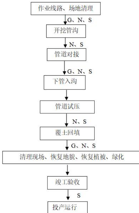
图 1.2-1 管线施工工艺流程
