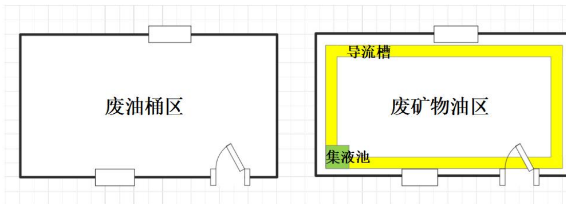
图 2.5-1 项目平面布置图（↑N）
