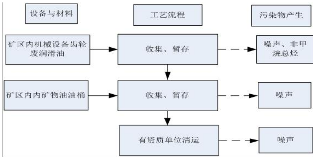
图 3.1.2-1 运营期工艺流程及产污环节
